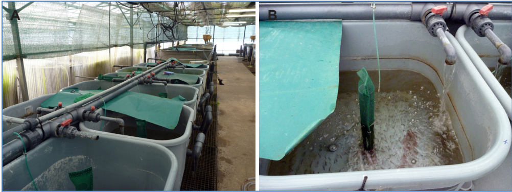
Figure 15. Bassins de 100 l installés dans un circuit recirculé, destinés à l'élevage larvaire du barbeau en conditions intensives (A); détail d'un bassin (B).
